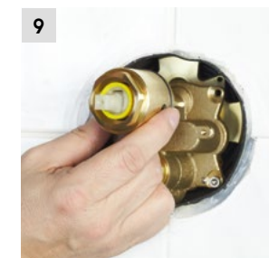
9 Montaż elementu funkcyjnego.
