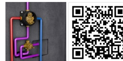
KLUDI - Montaż instalacji podtynkowej - natrysk Podtynkowa bateria wannowo-natryskowa z termostatem, głowicą natrysku, dyszami bocznymi i rączką natrysku
