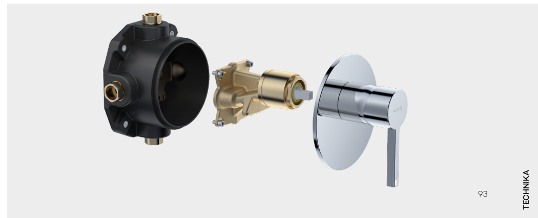
7 Montaż elementu funkcyjnego oraz zewnętrznego. Gotowe!
