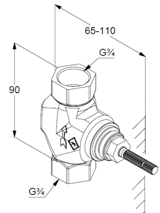
RYСУNEK Z WYMIARAMI
