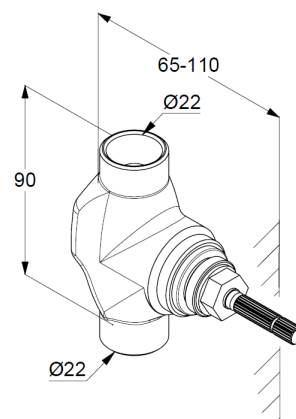
RYСУNEK Z WYMIARAMI
