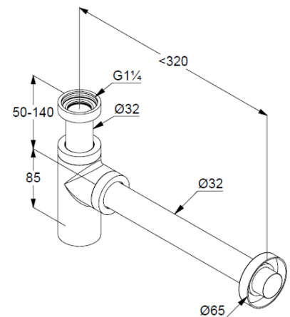
RYSUNEK Z WYMIARAMI
