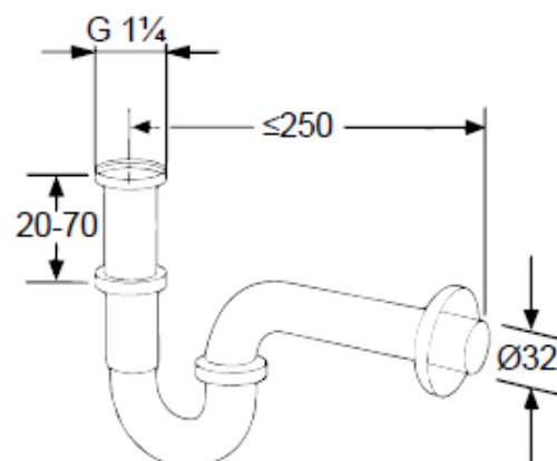
RYSUNEK Z WYMIARAMI
