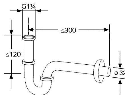
RYSUNEK Z WYMIARAMI
