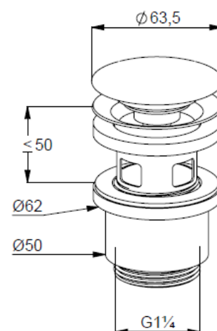
RYSUNEK Z WYMIARAMI
