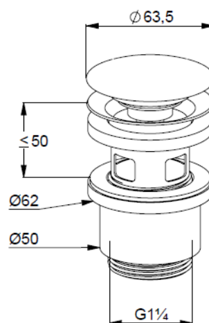
RYSUNEK Z WYMIARAMI
