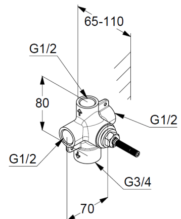
RYSUNEK Z WYMIARAMI
