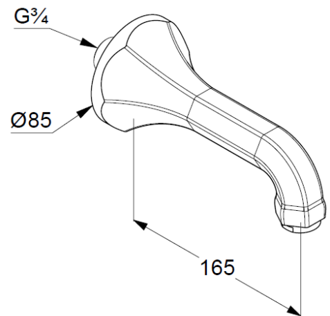
Rysunek techniczny
