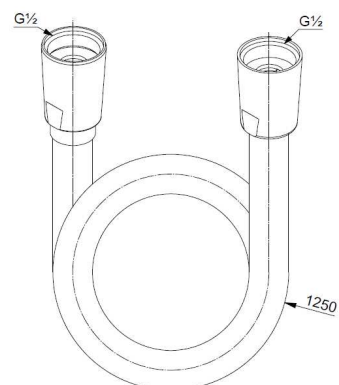
RYСУNEK Z WYMIARAMI
