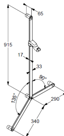
RYSUNEK Z WYMIARAMI
