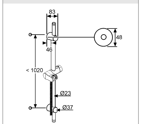
RYSUNEK Z WYMIARAMI
