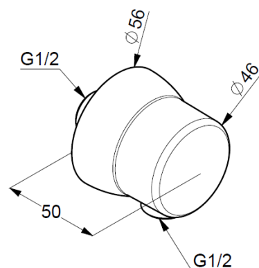
RYСУNEK Z WYMIARAMI
