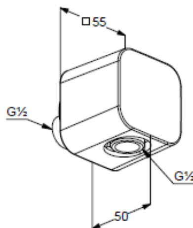
RYSUNEK Z WYMIARAMI
