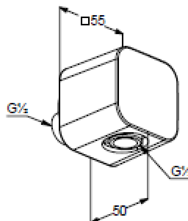
RYSUNEK Z WYMIARAMI
