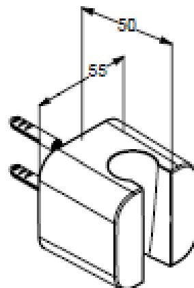
RYSUNEK Z WYMIARAMI
