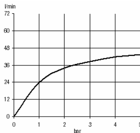
Diagram przepływu
