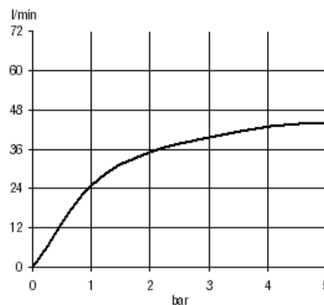
DIAGRAM PRZEPŁYWU
