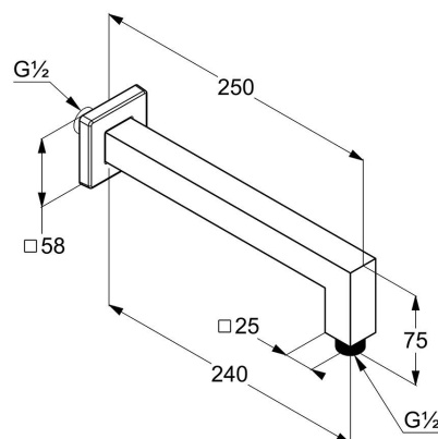
RYSUNEK Z WYMIARAMI
