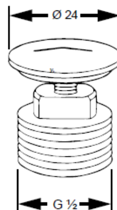
RYSUNEK Z WYMIARAMI
