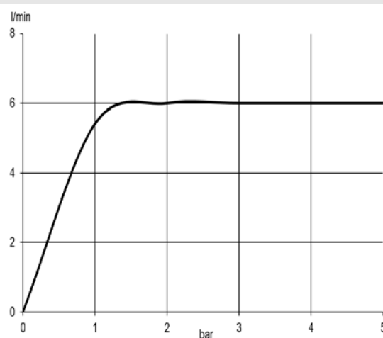
DIAGRAM PRZEPŁYWU
