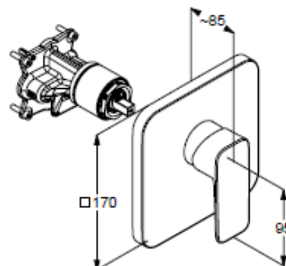
RYSUNEK Z WYMIARAMI
