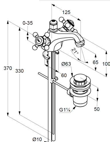
Rysunek techniczny
