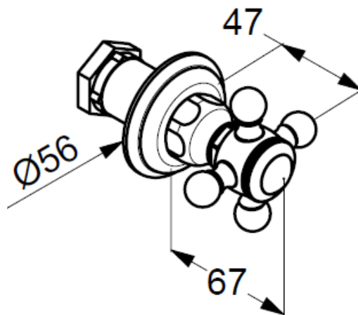
Rysunek techniczny
