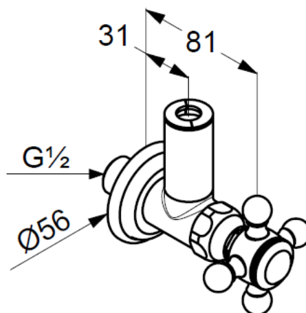
Rysunek techniczny
