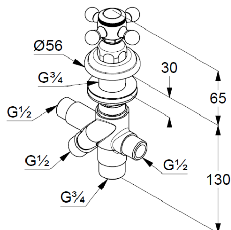
Rysunek techniczny
