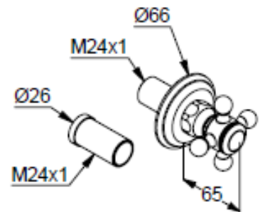
Rysunek techniczny
