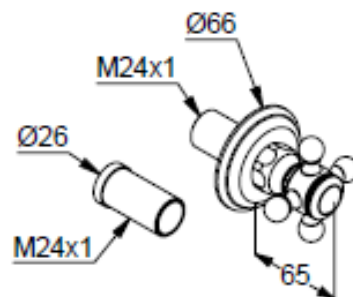
Rysunek techniczny
