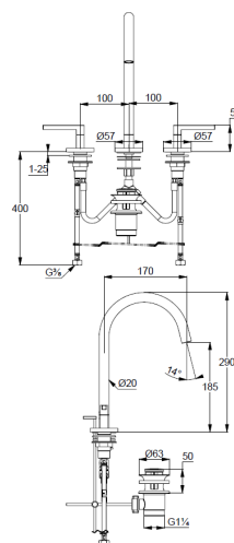
Maßzeichnung/ Dimensional drawing
