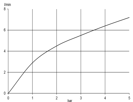
Durchfluss/ Flow rate
